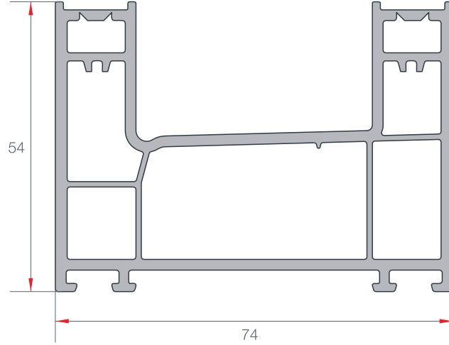
SÜRME KASA PROFİLİ SLIDING FRAME PROFILE EN 91 1.100 gr/m
