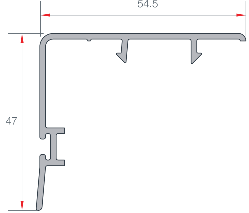
SÜRME KİLİT ADAPTÖRÜ SLIDING LOCK ADAPTER EN 99 0.285 gr/m
