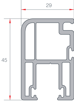
SÜRME SİNEKLİK KANAT PROFİLİ SLIDING FLY SCREEN SASH PROFILE EN 34 0.590 gr/m
