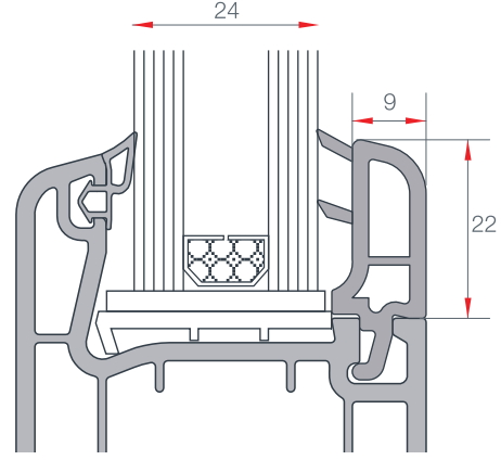
24 mm ÇİFT CAM ÇİTASI 24 mm DOUBLE GLAZING BEAD EN 109
