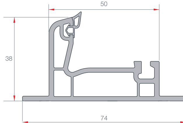
FİKS BAĞLANTI SLIDING FIX PROFILE EN 98 0.700 gr/m
