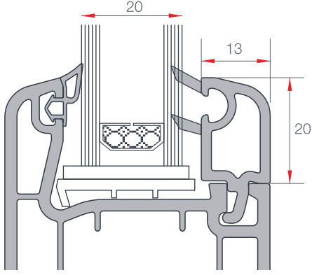
ÇİFT CAM ÇİTASI DOUBLE GLAZING BEAD EN 48
